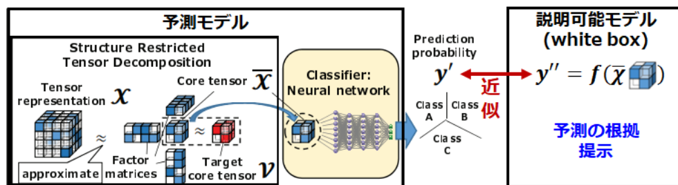
図3: DeepTensorの解析プロセス - 頂点間の関係の強さを要素とする行列・テンソル形式のデータから予測に必要とされる特徴が極力保持されるように重要成分と推定し、その成分を解釈することによって予測理由の説明を可能にするAI技術 (AAAI 2018. 3770-3077, 2018)
